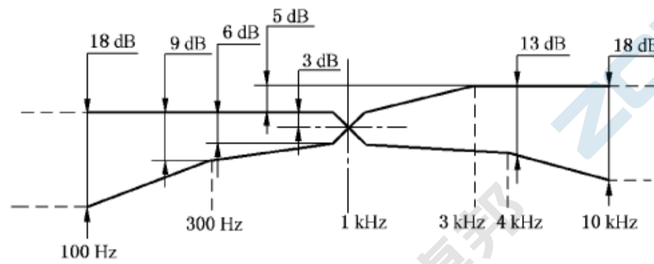
b) 指向性类型为单向、双向的传声器典型频响曲线容差范围
